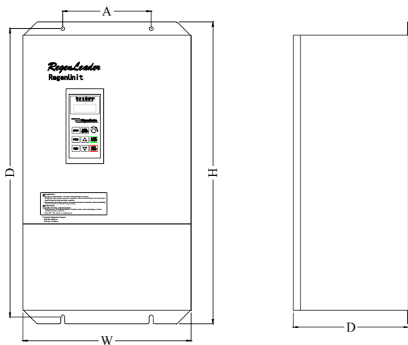
(图 2.4) RGU-F3/M3/T3 系列回馈装置的外形及尺寸
