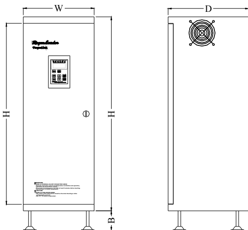
(图 2.3) RGU-LC3 系列回馈装置的外形及尺寸
