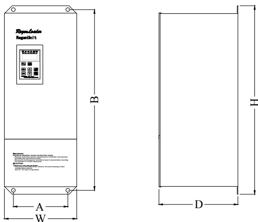
(图 2.2) RGU-N3/L3 系列回馈装置的外形尺寸
