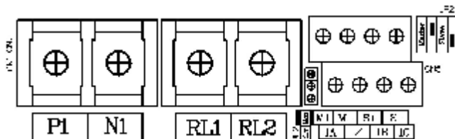
(图 3.1) BCM 系列小功率制动单元端子排列
