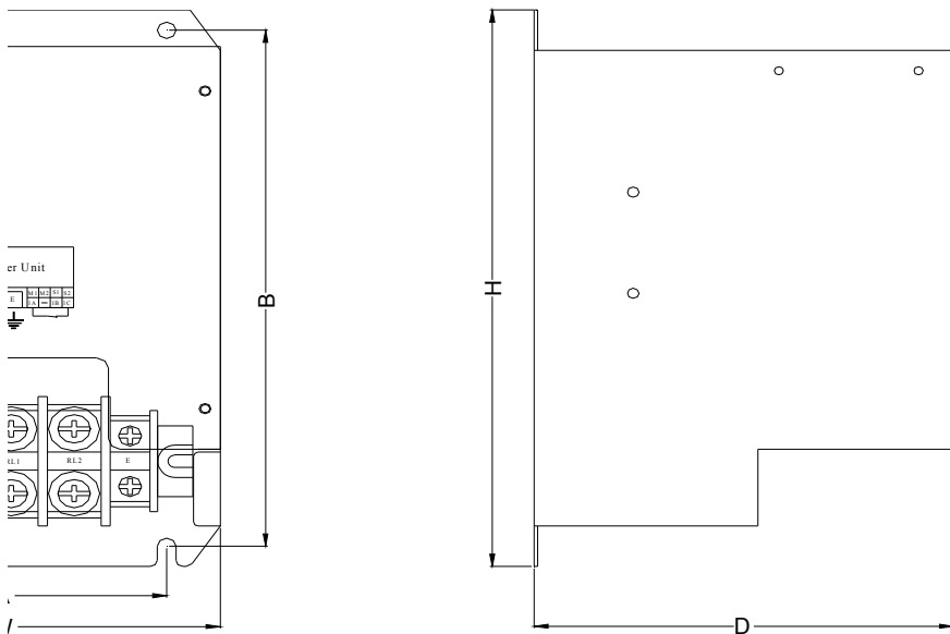
(图 2.4) BCM 系列制动单元的外形 C
