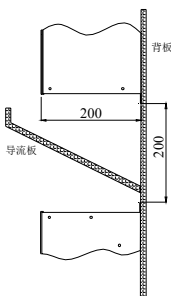
(3.6) 两台制动单元上下安装示意图
