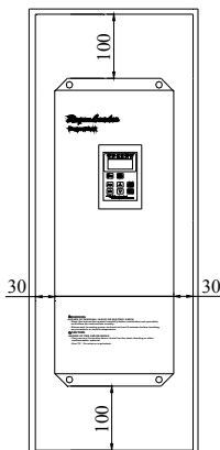
(图 3.5) BCM 系列制动单元的安装空间要求
