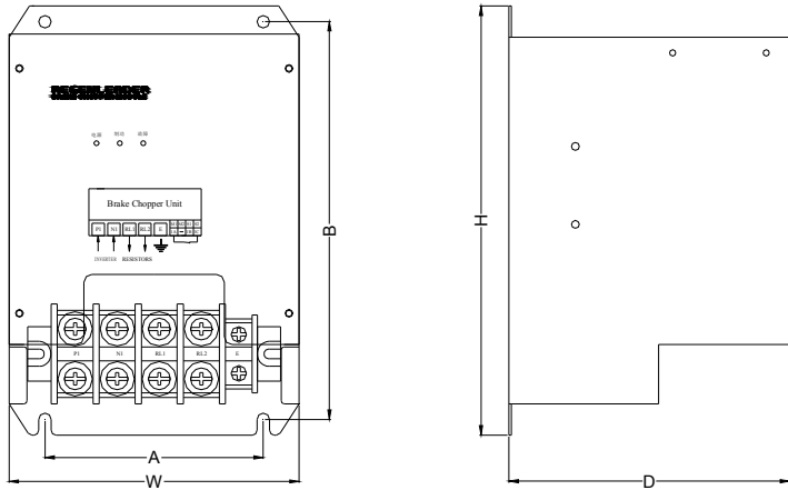
(图 2.3) BCM 系列制动单元的外形 B
