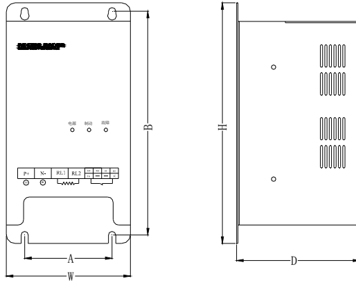
(图 2.2) BCM 系列制动单元的外形 A
